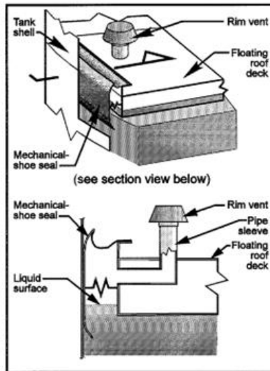
Rim Vent
